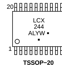
TSSOP-20
