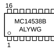
SOEIAJ-16
