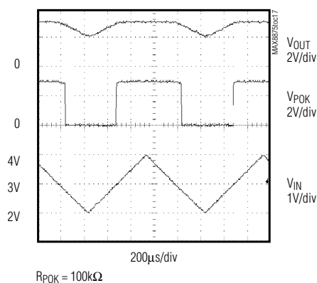
POK OUTPUT
