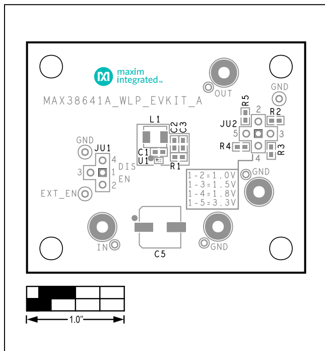
MAX38641A WLP EV Kit—Top Silkscreen
