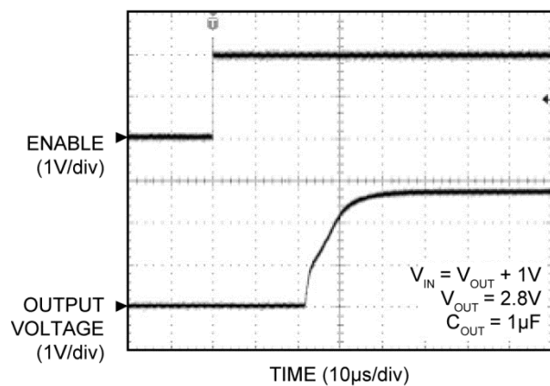
Enable Turn-On
