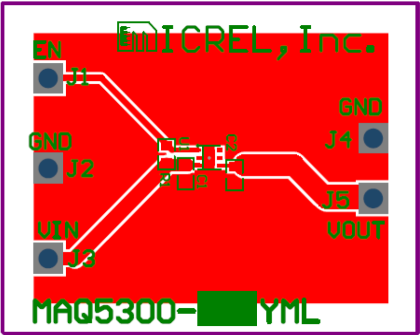
Top Layer
