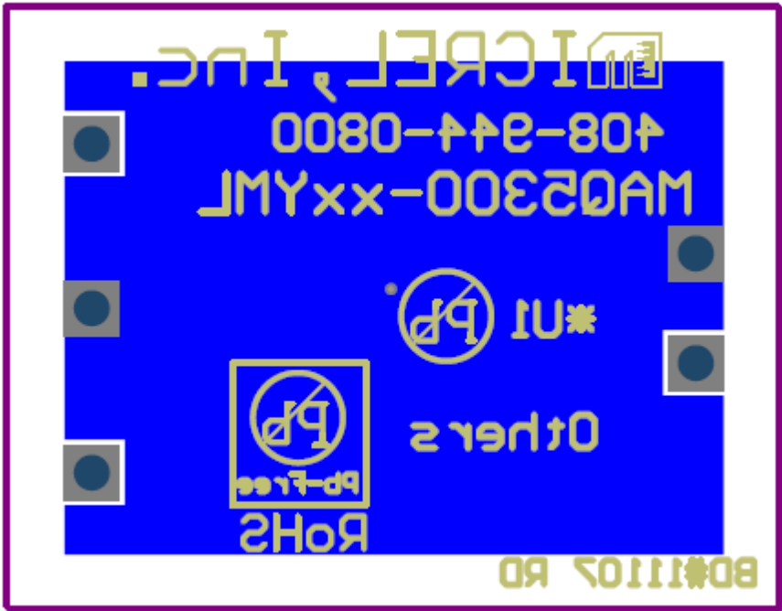
Bottom Layer
