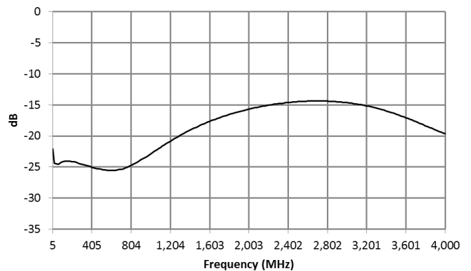
Output Return Loss (pin2)
