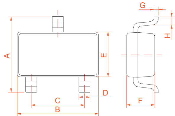
SOT-23-3L
