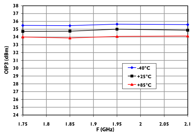
OIP3
