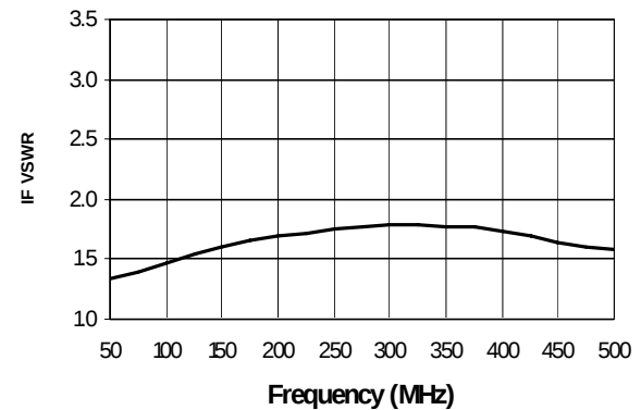
IF VSWR
