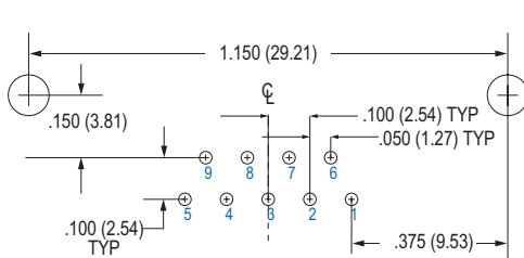
9 PIN M83513/16-A
