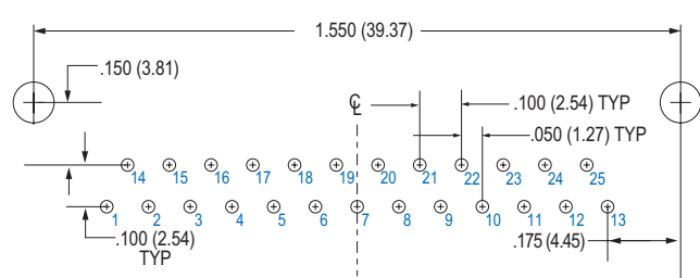
25 SOCKET M83513/19-D
