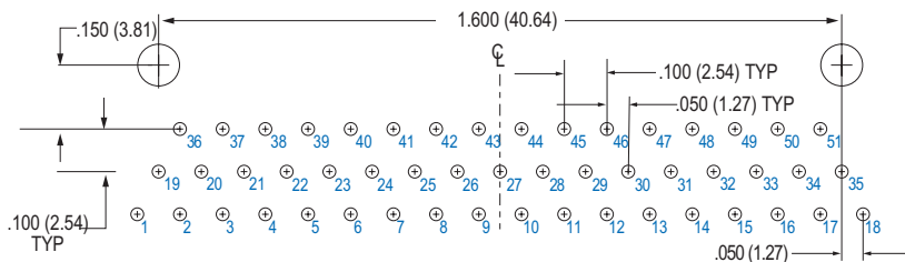
51 SOCKET M83513/20-G
