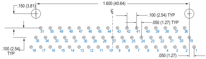
51 PIN M83513/17-G
