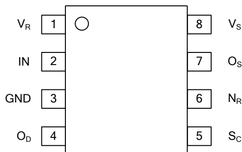
DIP-8 / SOP-8
