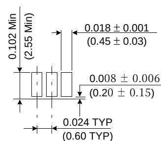
Detail Y
