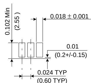
Detail Y
