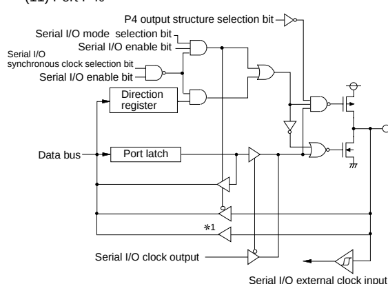
(11) Port P46
