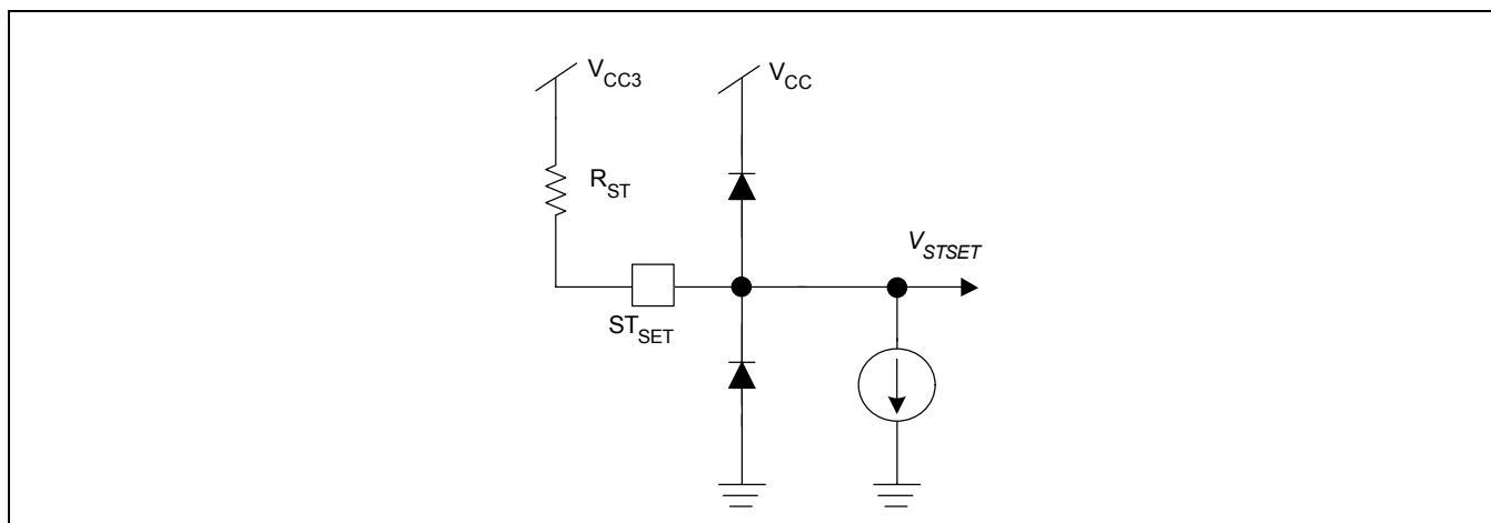
Figure 3-5. STset Input
