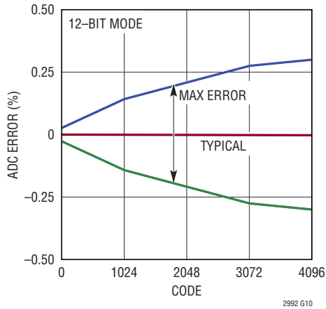
ADC Error (GPIO)
