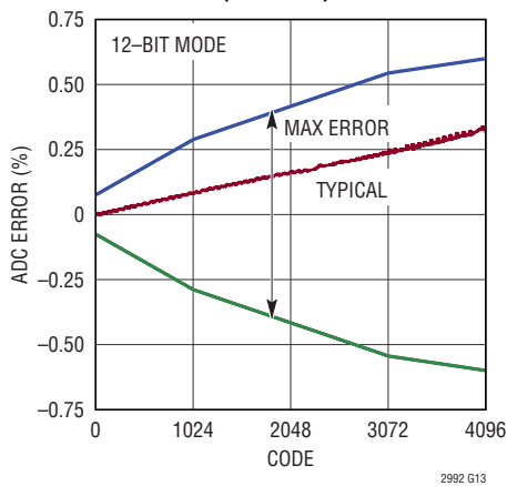
ADC Error ( \Delta SENSE)
