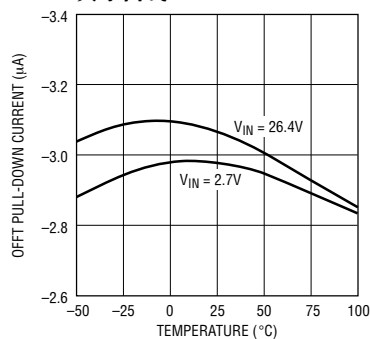
OFFT 下拉电流与温度的关系曲线
