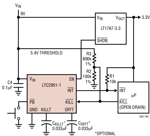
图5：采用 \overline{\text{KILL}} 输入来进行输入电压监视
