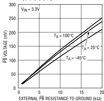
\overline{\text{PB}} 电压与外部接地 \overline{\text{PB}} 电阻的关系曲线
