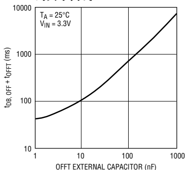
关断反跳时间 ( t_{DB, OFF} + t_{OFFT} ) 与 OFFT 外部电容器的关系曲线
