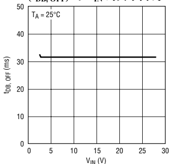
内部缺省关断反跳时间 ( t_{DB, OFF} ) 与 V_{IN} 的关系曲线
