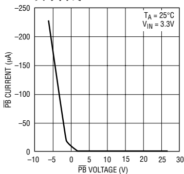
\overline{\text{PB}} 电流与 \overline{\text{PB}} 电压的关系曲线
