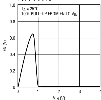
\overline{\text{EN}} (LTC2951-1) 电压与 V_{IN} 的关系曲线
