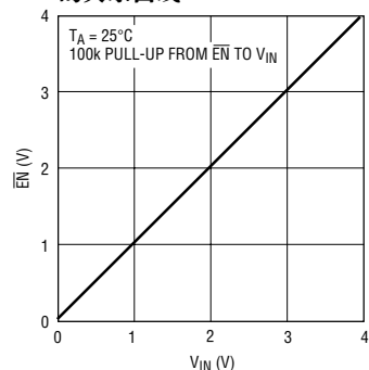
\overline{\text{EN}} (LTC2951-2) 电压与 V_{IN} 的关系曲线
