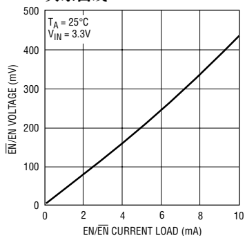
\overline{\text{EN}}/\overline{\text{EN}} V_{OL} 与电流负载的关系曲线
