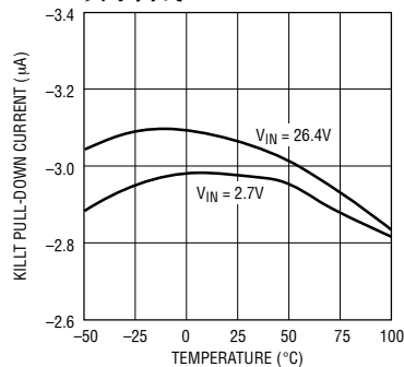
KILLT 下拉电流与温度的关系曲线
