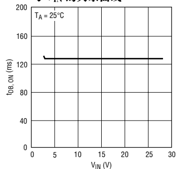
接通反跳时间 ( t_{DB, ON} ) 与 V_{IN} 的关系曲线
