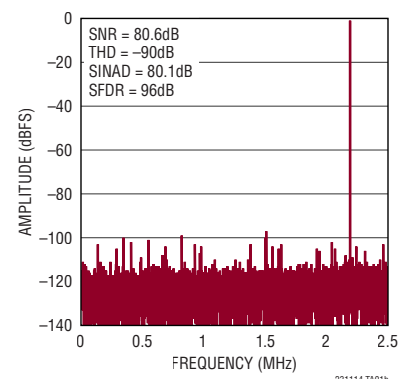
32k Point FFT f_{\text{SAMPL}} = 5\text{Mps} , f_{\text{IN}} = 2.2\text{MHz}
