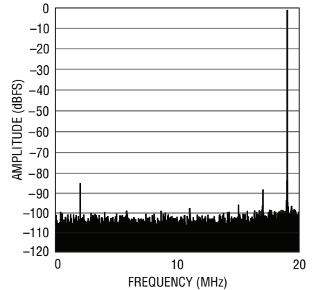
LTC2264-14: 8k Point FFT, f_{IN} = 139\text{MHz} , -1\text{dBFS} , 40\text{Mps}
