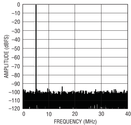
LTC2259-12: 8k Point FFT, f_{IN} = 5\text{MHz} , -1\text{dBFS} , 80\text{Mpsps}
