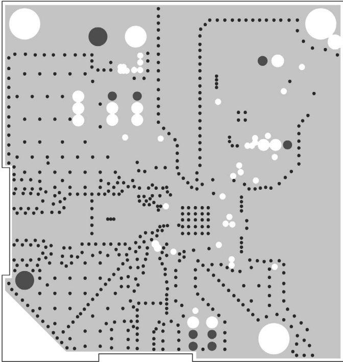
Inner Layer 3
