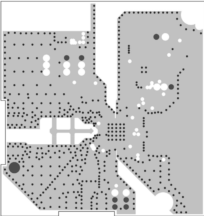
Inner Layer 2
