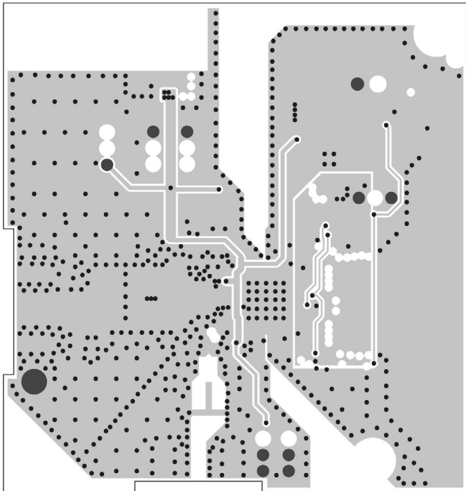
Inner Layer 5
