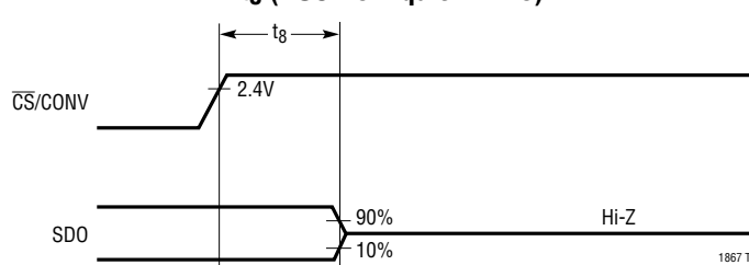
t 8 (BUS Relinquish Time)
