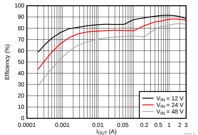
效率与输出电流间的关系 ( V_{\text{out}} = 5\text{V} , f_{\text{sw}} = 500\text{kHz} )
