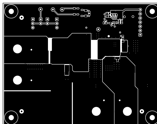
Figure 24. Top Layer
