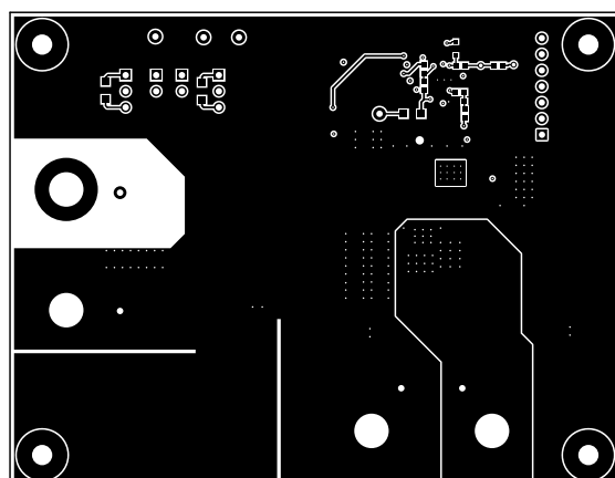
Figure 27. Bottom Layer
