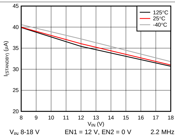
Figure 4. I_{\text{STANDBY}} vs VIN
