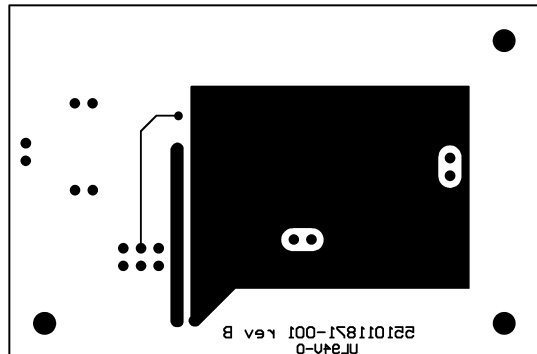
Bottom Layer
