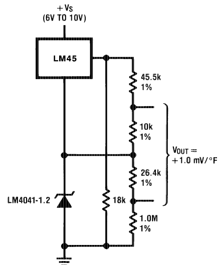
FIGURE 8. Fahrenheit Thermometer
