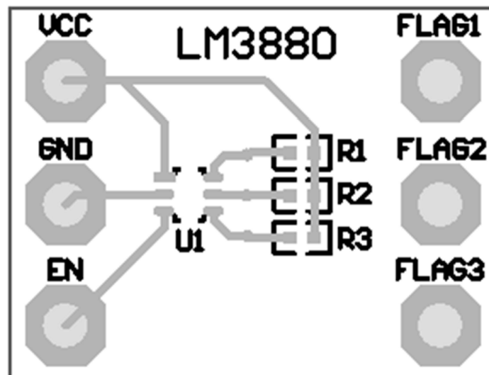
Figure 20. LM3880 Top
