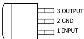
TO-263 3L
