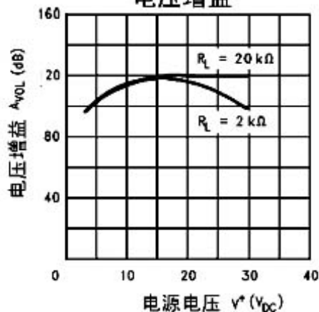
电压增益
