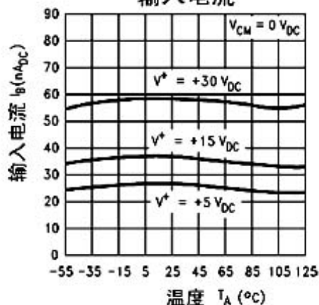
输入电流
