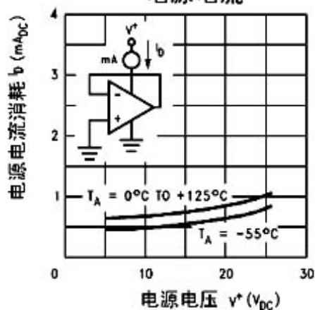
电源电流
