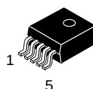
D 2 PAK D2T SUFFIX CASE 936A
