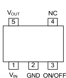
SOT-25
