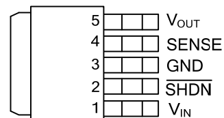
TO-263-5
