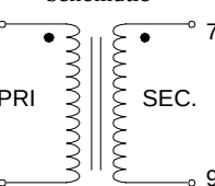
T-30402 & 30403 Schematic
