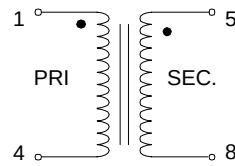
T-30404 & 30405 Schematic
