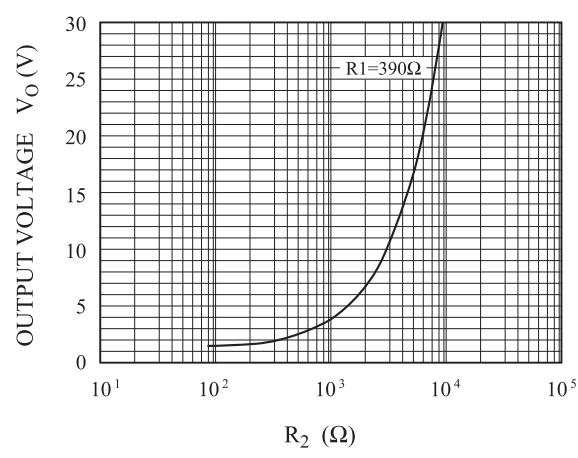
Fig. 10 R_2 - V_O
