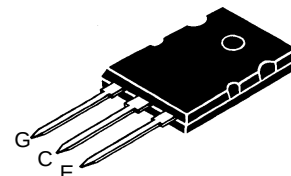
TO-264 (IXSK)
