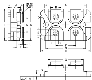
SOT-227B miniBLOC
