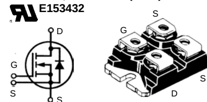
miniBLOC, SOT-227 B (IXFN)
