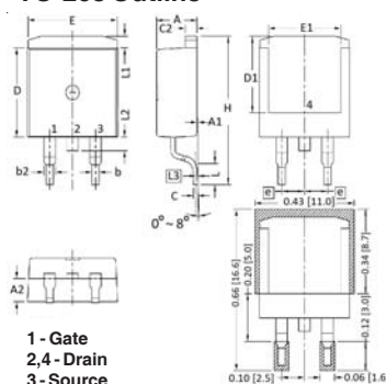
TO-263 Outline
