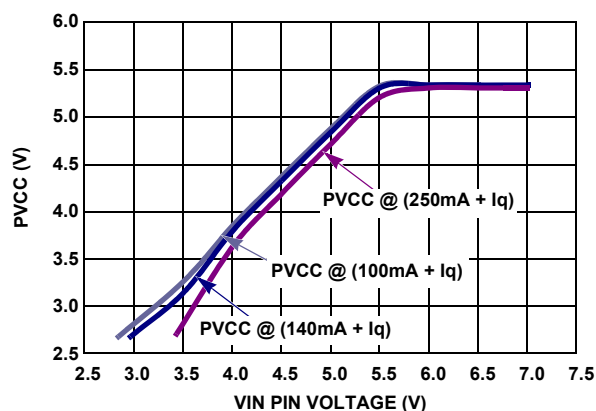
FIGURE 27. PVCC vs VIN VOLTAGE
