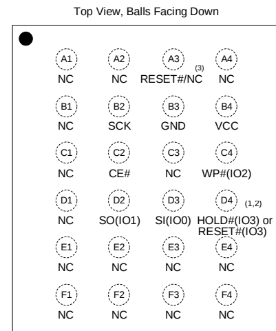
24-ball TFBGA 6x8mm
