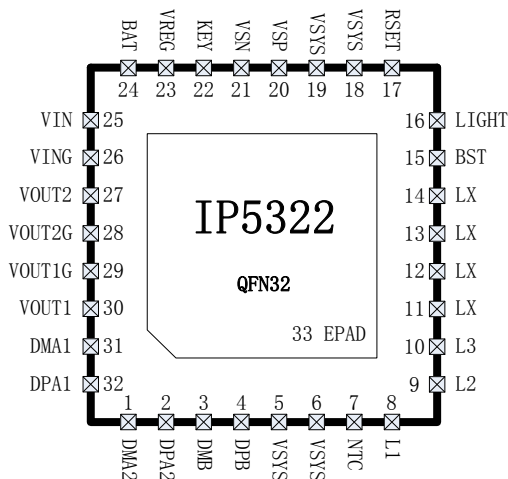
图 2 IP5322 引脚图
