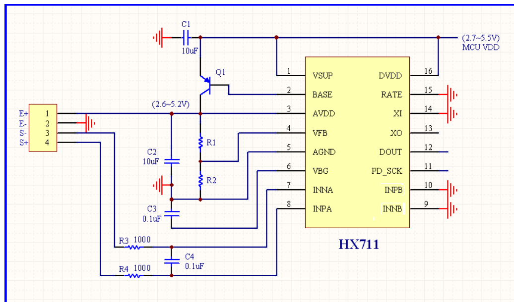
图五 HX711 称重衡器应用参考设计线路图之二
