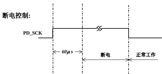
图三 断电控制
