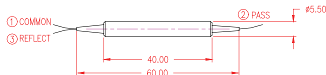
P2: 900 \mu m loose tube
