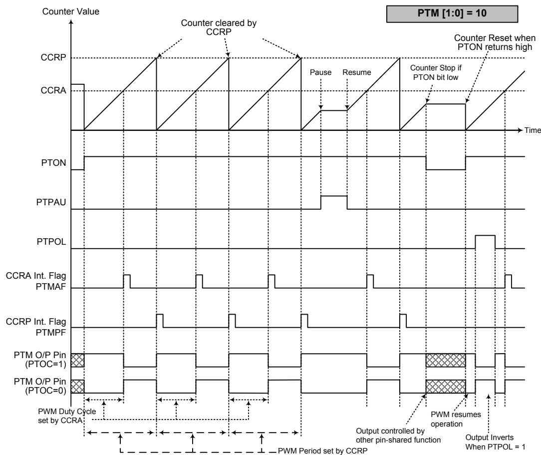
PWM Output Mode
