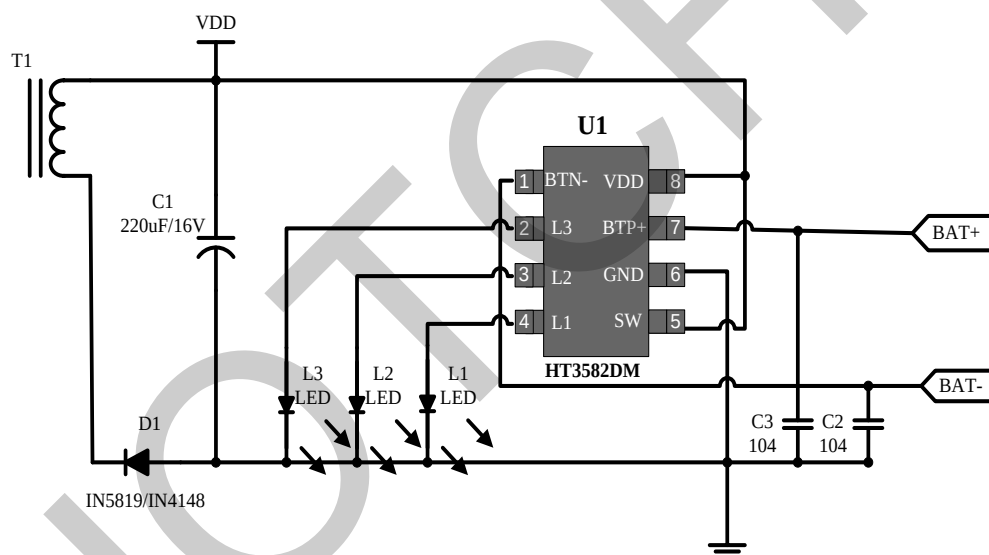
图 4.1 HT3582DM 普通 3 灯应用方案（如将 L3 去掉，则为普通二灯模式）
