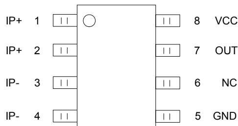
SOP8 封装
