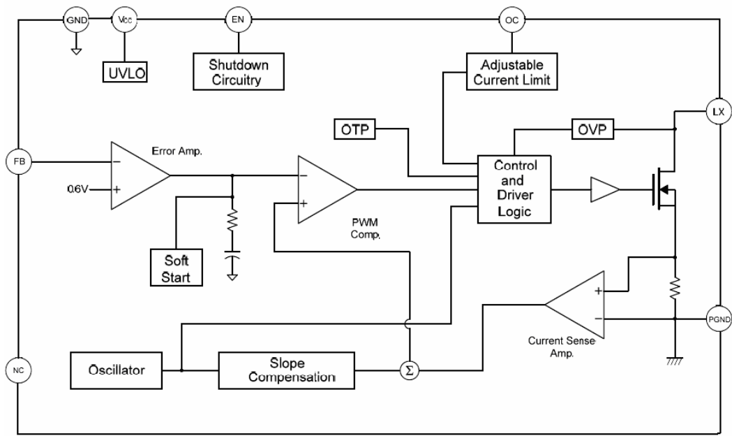
图 3 功能框图
