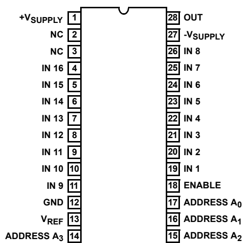
HI-546 (CERDIP, PDIP, SOIC)
