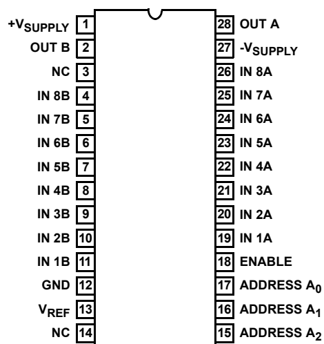
HI-547 (CERDIP, PDIP, SOIC)
