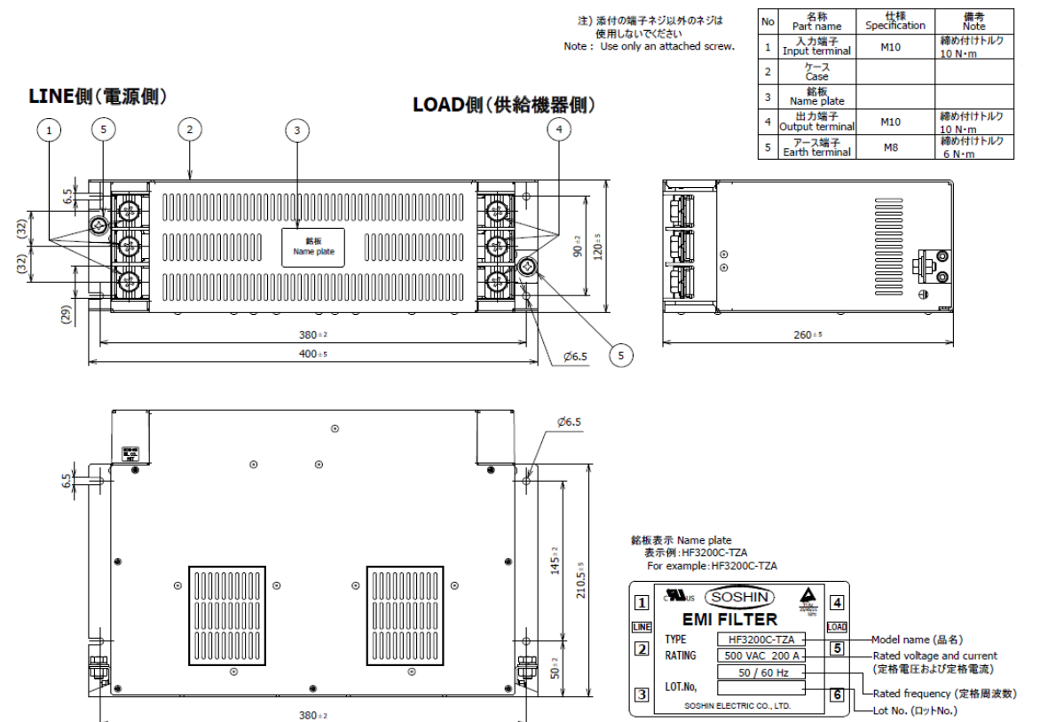
fig.3 (200~300A)
