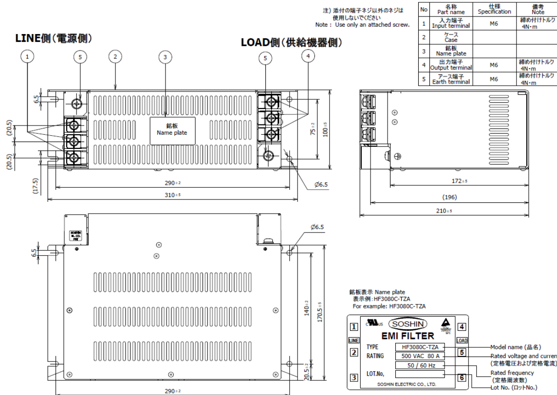
fig.1 (80~100A)
