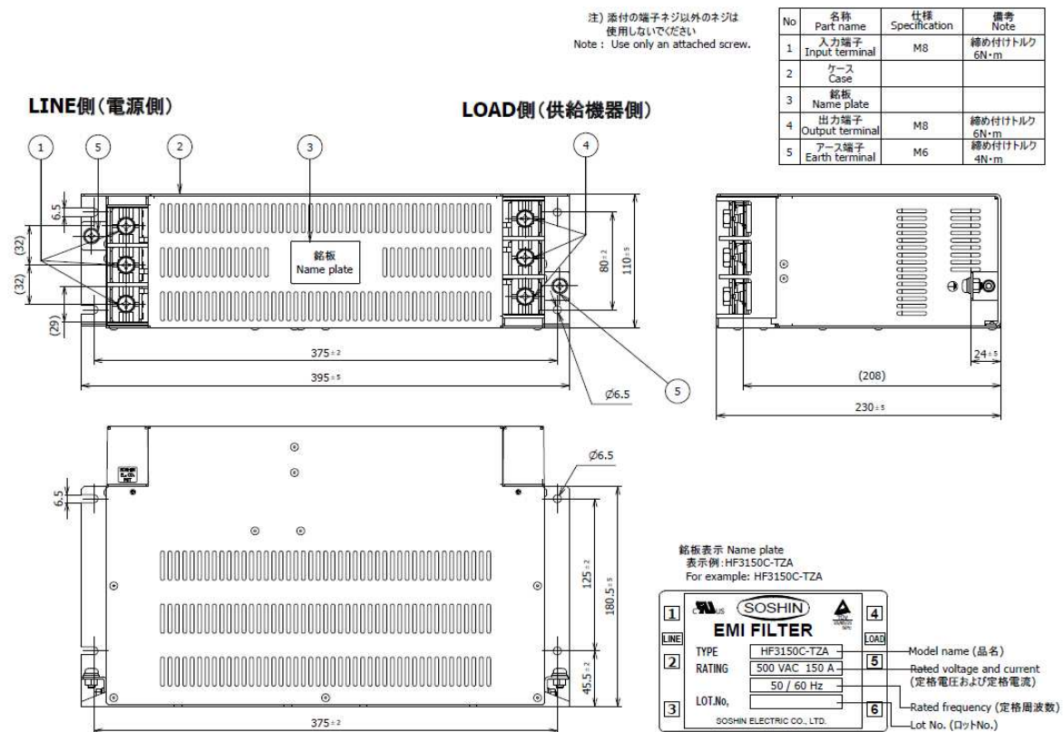
fig.2 (150A)
