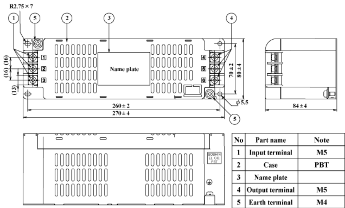
fig.2 (40-60A)
