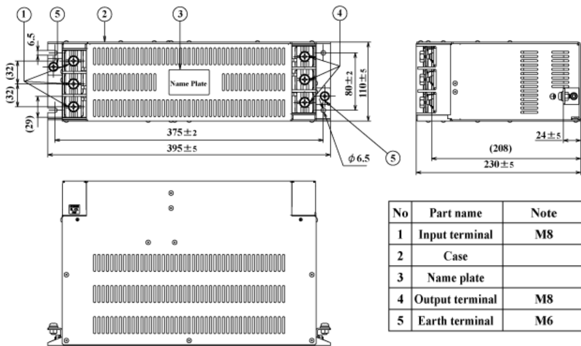
fig.4 (150A)
